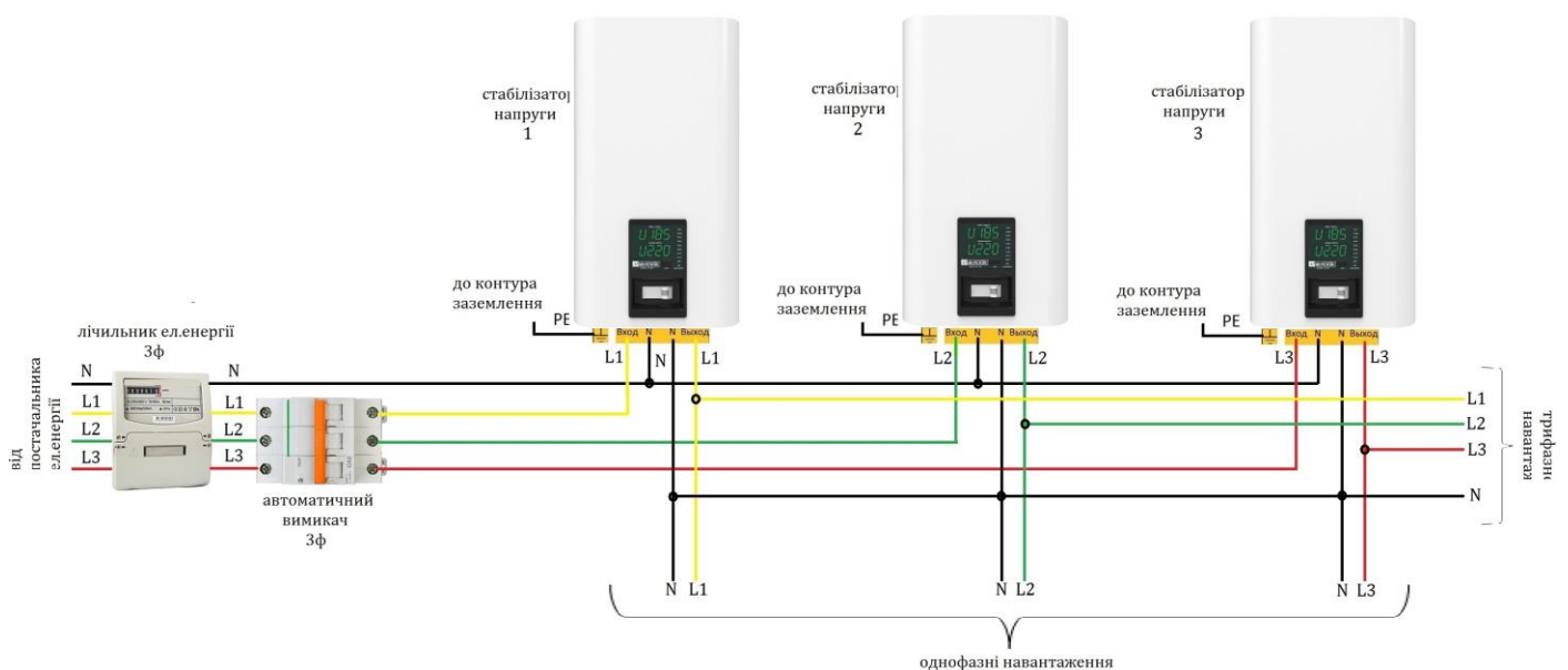
Рисунок 8. Схема підключення стабілізатора до трифазної мережі
