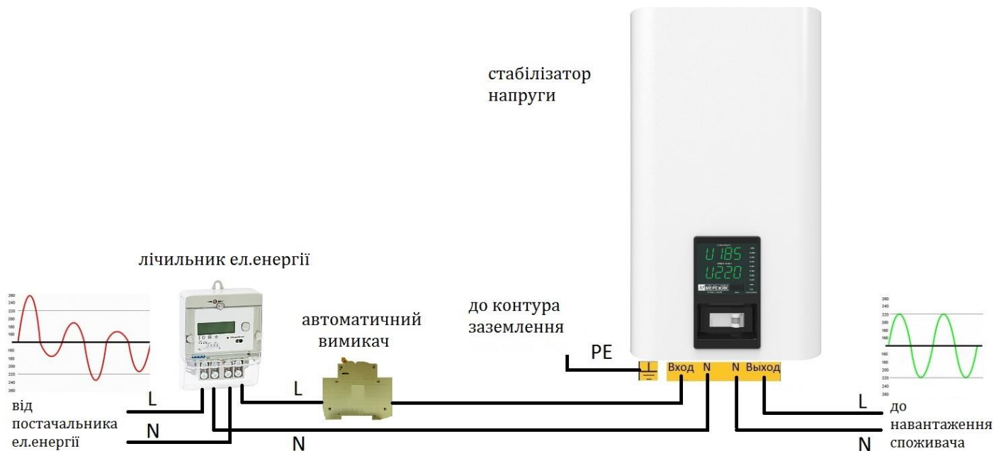
Рисунок 7. Схема підключення стабілізатора до однофазної мережі
