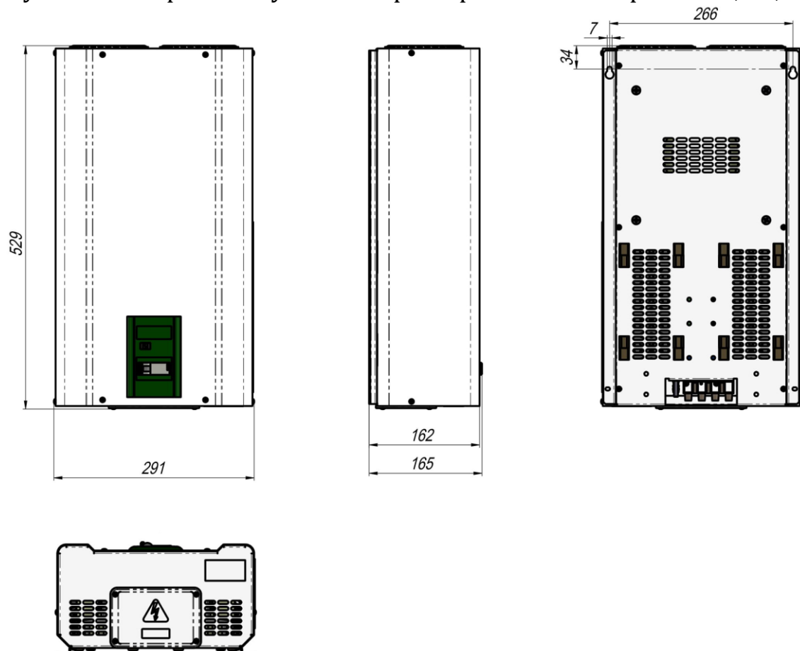
Рисунок 5. Габаритні та установчі розміри стабілізаторів на 50, 63, 80А
