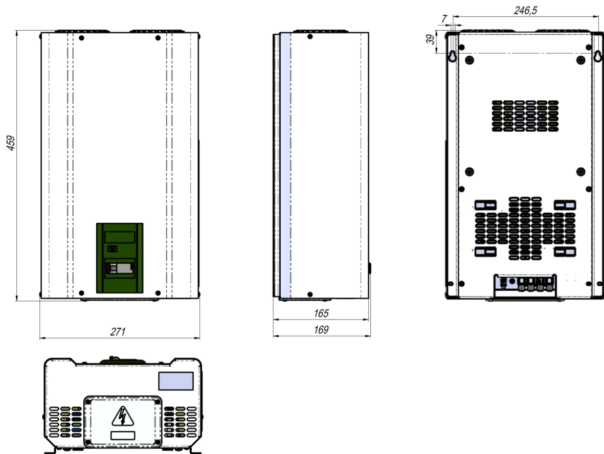
Рисунок 4. Габаритні та установчі розміри стабілізаторів на 25, 32, 40А
